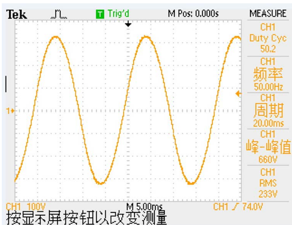
图 3: 输出波形
